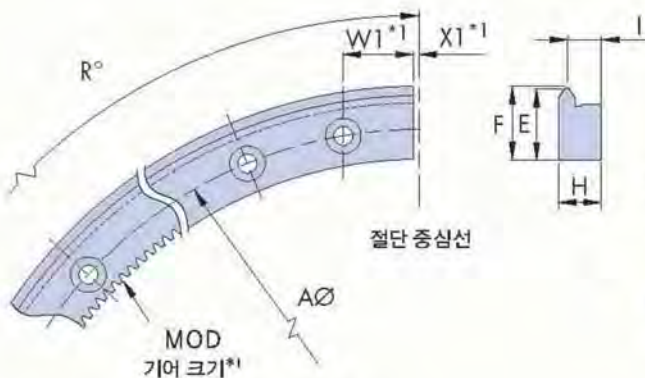
외부 싱글 에지 트랙 세그먼트 - TRE
