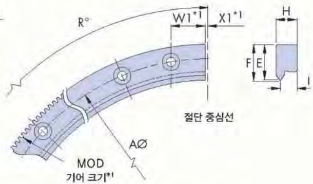
내부 싱글 에지 트랙 세그먼트 - TRI
